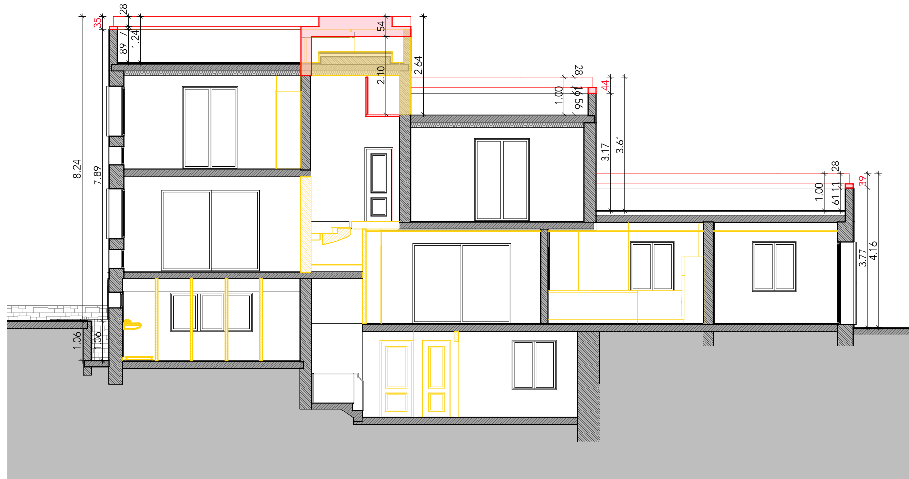
Principe de mise aux normes avec garde-corps en verre + maçonnerie
