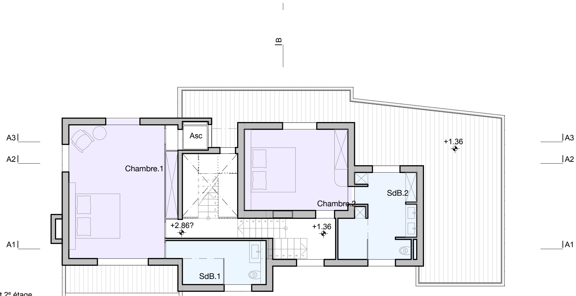
Plan du 1 er et 2 e étage
